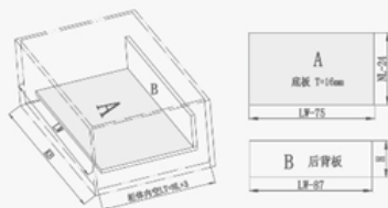
后背板裁板尺寸
