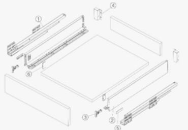
COMPONENTS | 组件
