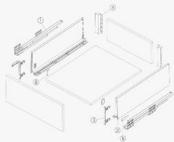
COMPONENTS | 组件
