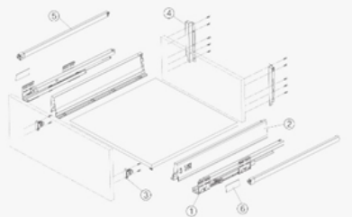
COMPONENTS | 组件
