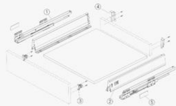
COMPONENTS | 组件
