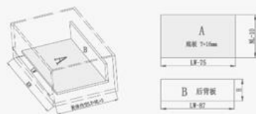
后背板裁板尺寸
