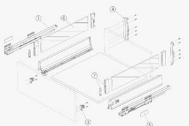
COMPONENTS | 组件
