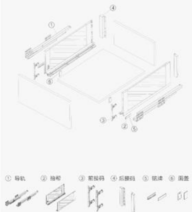
COMPONENTS | 组件
