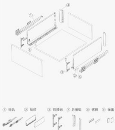
COMPONENTS | 组件
