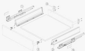
COMPONENTS | 组件
