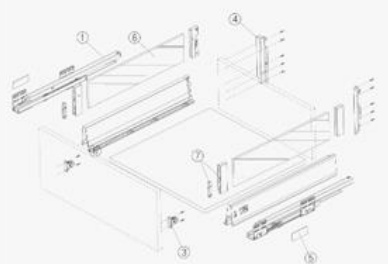
COMPONENTS | 组件
