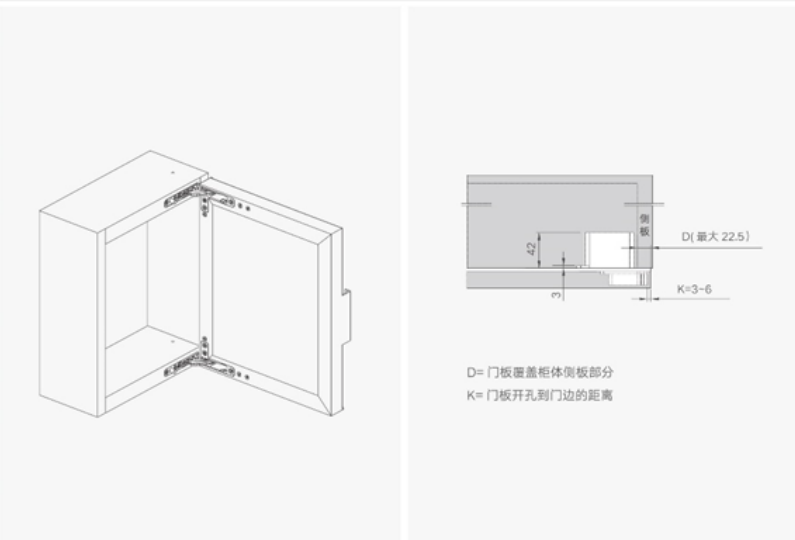
INSTALLATION SIZE | 安装尺寸 (A=B)
