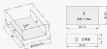
后背板裁板尺寸
