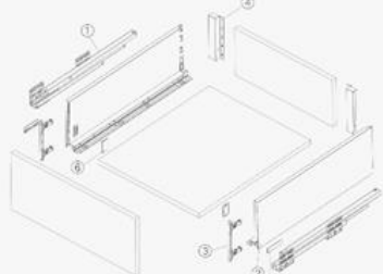
COMPONENTS | 组件
