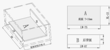
后背板裁板尺寸
